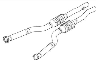
Abbildung: 20 Teilenummer (AWRON): -- Teilenummer (BMW): 18 30 7 835 520, 18 30 7 835 519
