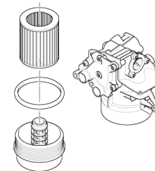
Abbildung: 14 Teilenummer (AWRON): -- Teilenummer (BMW): 11 42 7 837 710
